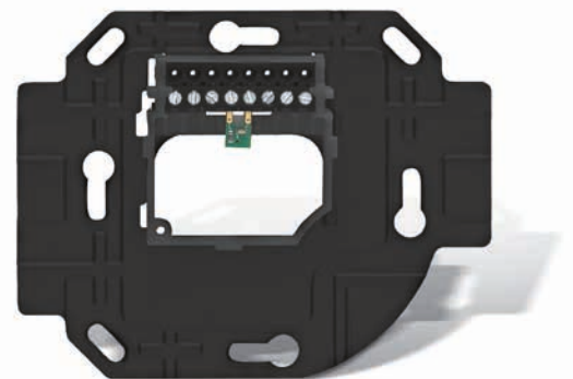
Montageplatte REH117X für Innensprechstelle elcom.touch und elcom.fon.
